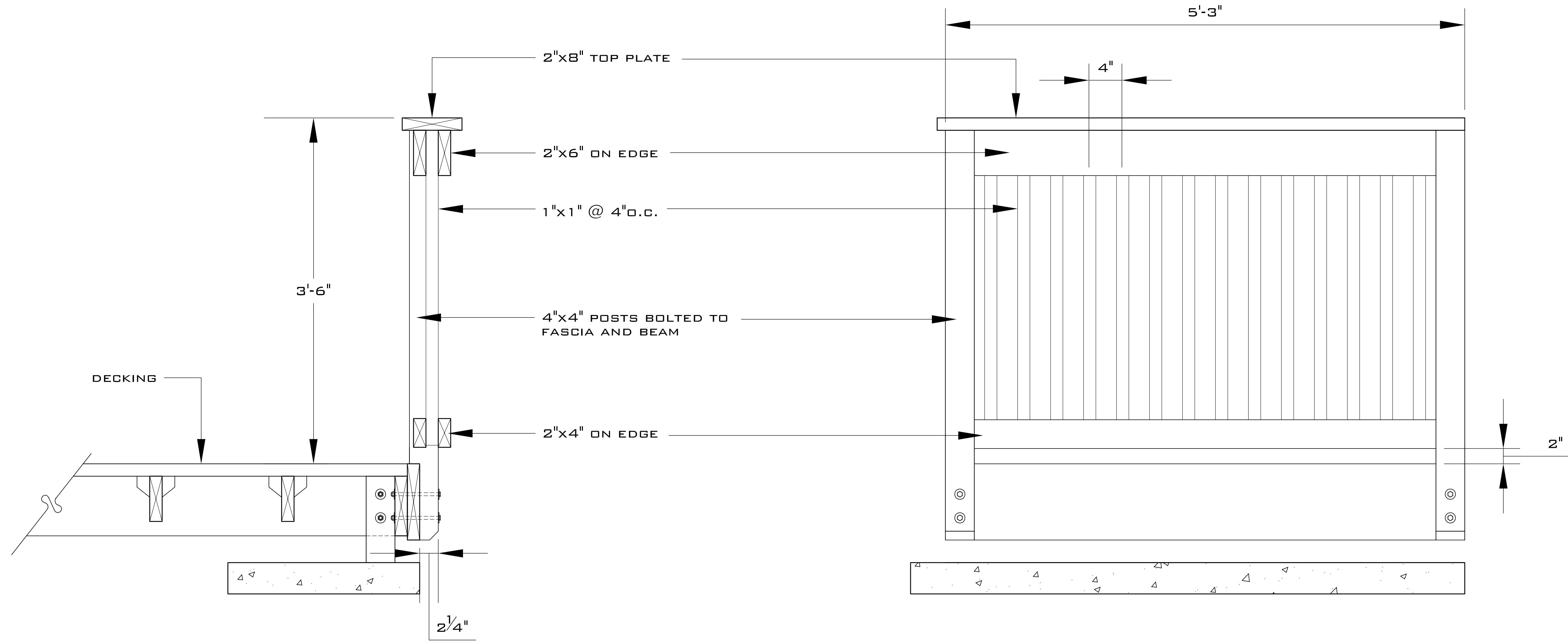
2 SECTION SCALE: 1 1/2" = 1'-0"
